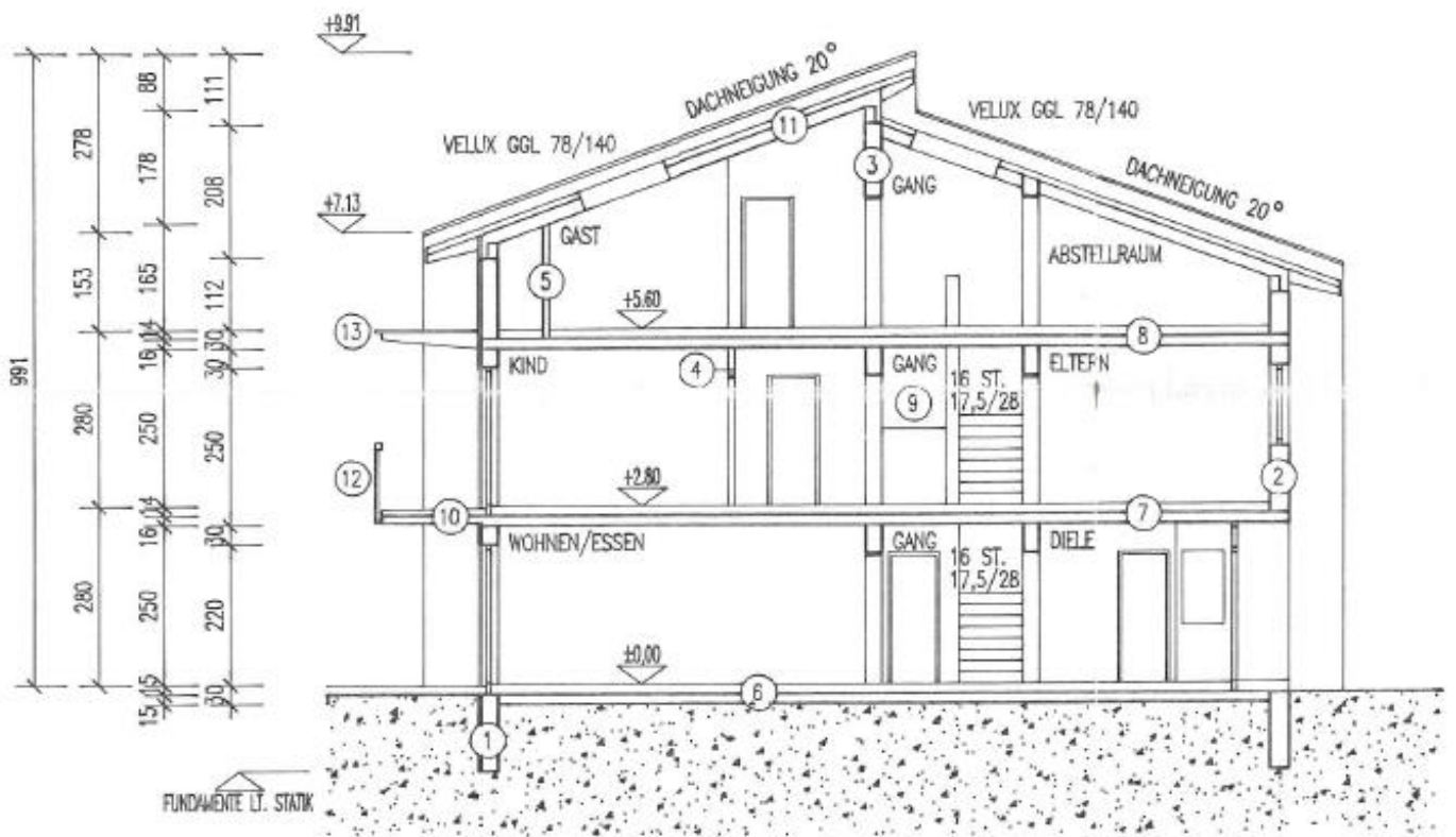
SCHNITT A-A
